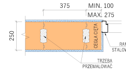
- WIĄZANIE PRZY OKŁADZINIE DRZWI, 2. RZĄD MURÓW
