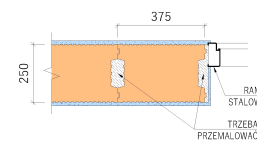
- WIĄZANIE PRZY OKŁADZINIE DRZWI, 1. RZĄD MURÓW
