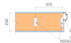
- WIĄZANIE PRZY OKŁADZINIE DRZWI, 1. RZĄD MURÓW
