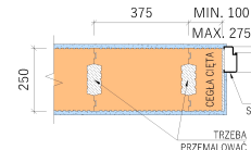
- WIĄZANIE PRZY OKŁADZINIE DRZWI, 2. RZĄD MURÓW
