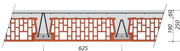
Grubość stropu 250 mm
