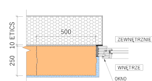
- WIĄZANIE PRZY OKŁADZINIE OKIENNEJ, 1. RZĄD MURÓW
