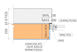
- WIĄZANIE PRZY OKŁADZINIE OKIENNEJ, 2. RZĄD MURÓW
